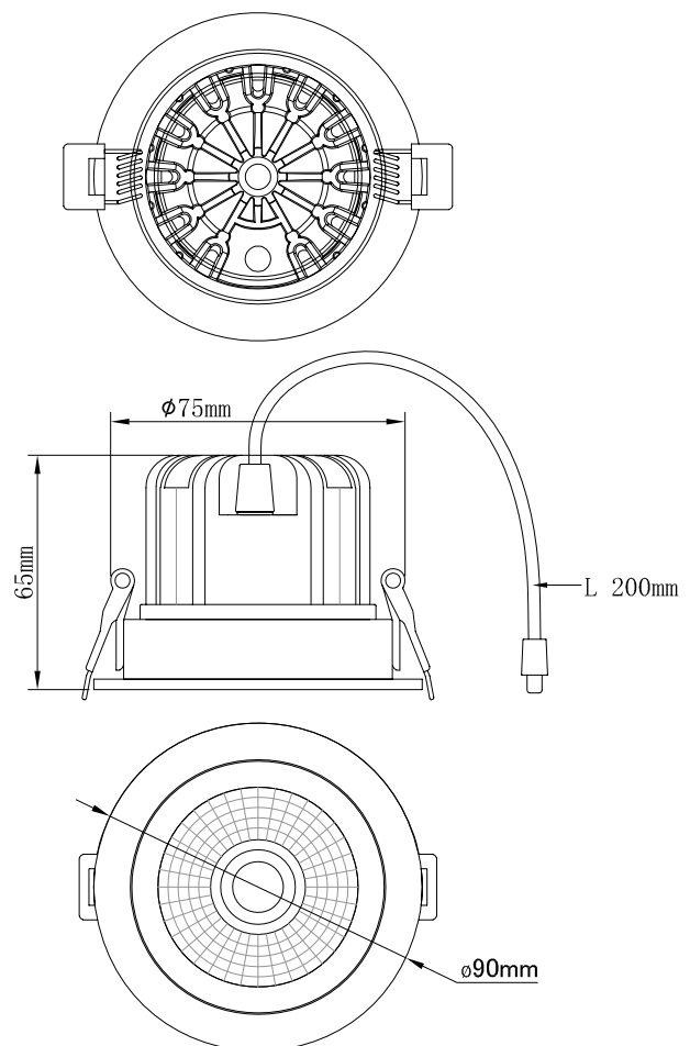
Abb. 2: Abmessungen
