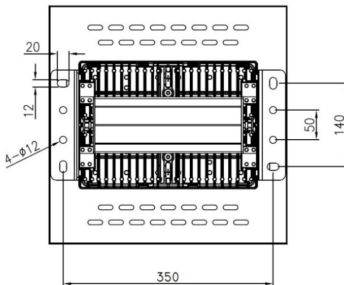
Abb. 2: Befestigungspunkte der Montagebügel
