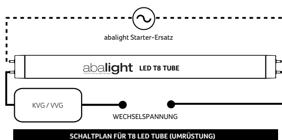
Abb. 2: elektrische Schaltpläne
