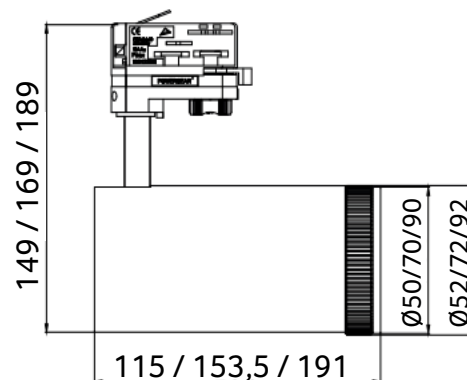
Produktabmessungen
