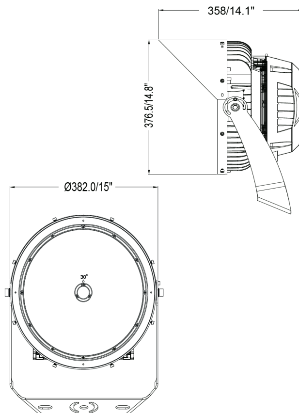
Abb. 2: Abmessungen Außenleuchte ERANA
